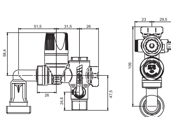
NA53M2 - modèle coudé
