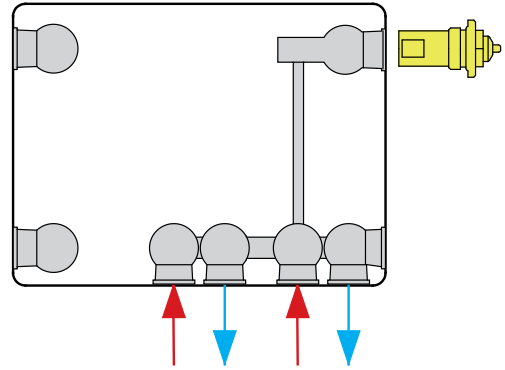
Vues: face avant
